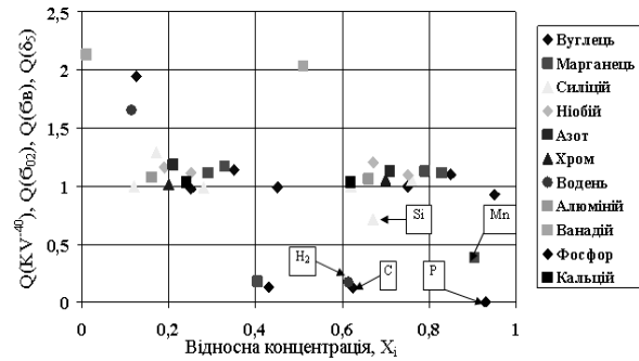
Рис. 3. Вплив вмісту елементів на всі критерії якості сталі E36
