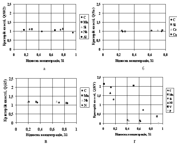
Рис. 2. Вплив вмісту елементів на окремі критерії якості прокату сталі E36
