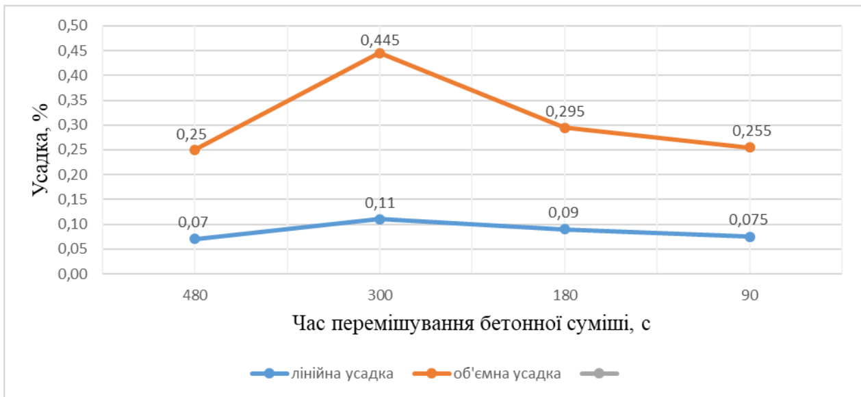
Рис. Залежність лінійної та об'ємної усадки бетонів від часу перемішування бетонної суміші
