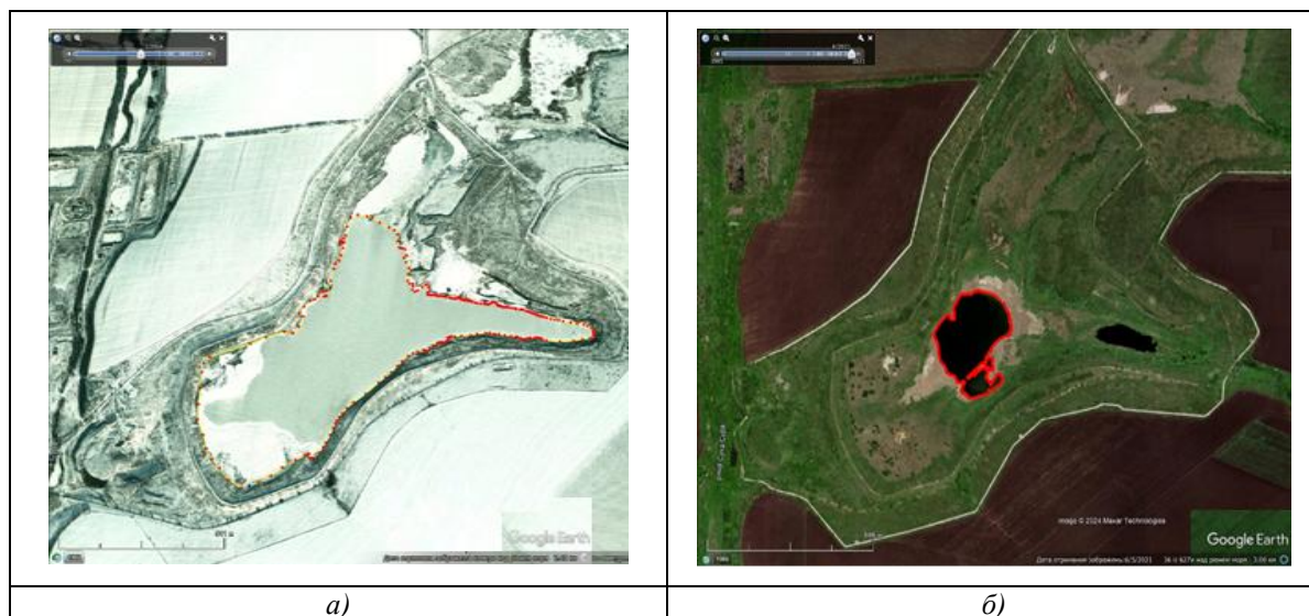
Рис. 1. Фото загального виду на хвостосховище «Сухачівське» секція II Червоним кольором позначено фактичний контур «дзеркала» на карті а) фото зроблено 23.02.2004 р. ( Google Earth Pro ); б) фото зробленого 08.07.2022 р. ( Google Earth Pro ). Виміри для ізоліній (сітки рельєфу) зроблені 25.09.2023 р.
