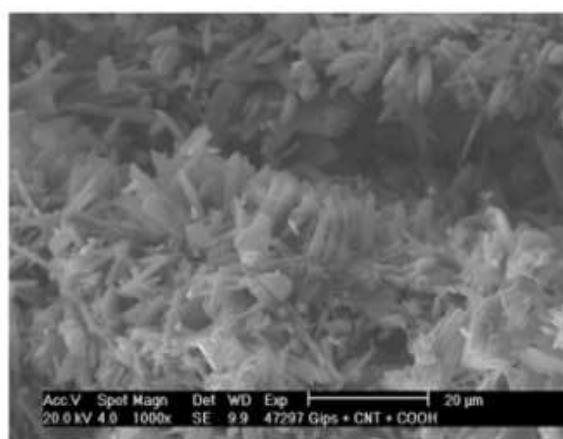
Рис. 4. Микрофотографии гипсовой композиции:
