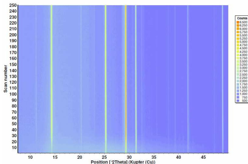
Рис. 2. Інтенсивність в процесі гідратації напівводного гіпсу з добавкою пластифікатора полікарбоксилата П-11
