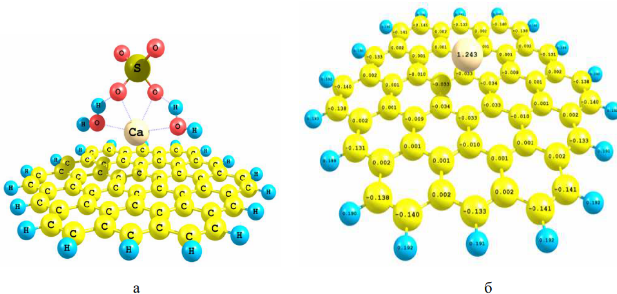
Рис. 5. Модельные фрагменты поверхности УНТ, взаимодействующие: с молекулой гипса (а); ионом \text{Ca}^{2+} (б)
