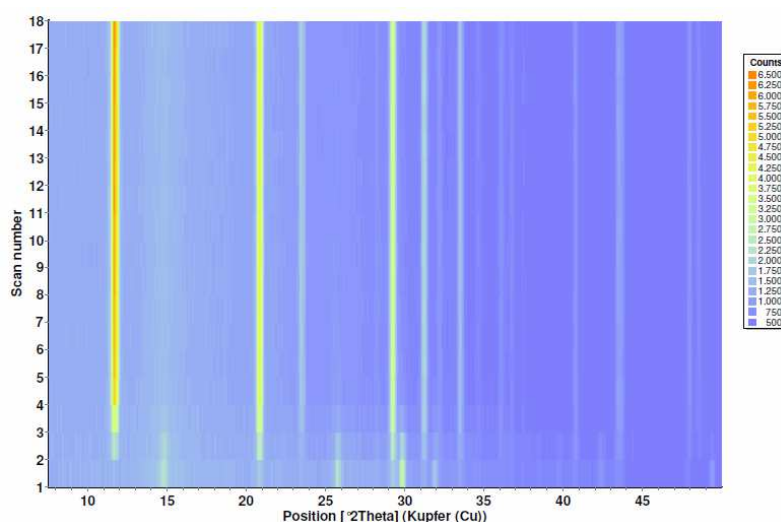
Рис. 3. Інтенсивність в процесі гідратації напівводного гіпсу з добавкою пластифікатора полікарбоксилата П-11, модифіцированного УНТ
