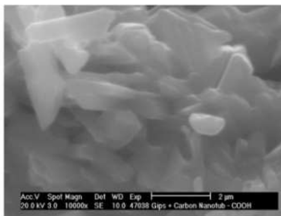
Рис. 4. Микрофотографии гипсовой композиции:
