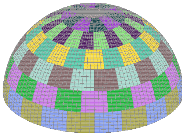
Рис. 4 – Схема разбивки конструкции опалубки на модульные составные элементы
