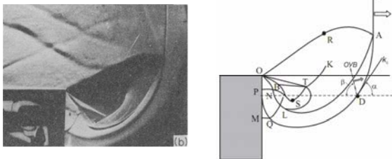
Рис. 5. Теплеровское фото (а) и схема течения при дифракции сильной ударной воздушной волны на прямом угле (б): IA – падающая ударная волна, AM – дифрагированная ударная волна, AO – отраженная акустическая волна, AL – контактная поверхность, TS – волна торможения, OS – линия отрыва, TB – косая ударная волна, TK – вторичный скачок, NP – пристеночный скачок, Q – тройная точка, R и D – точки искривления фронта [11] / The Tepler photo (a) and the flow pattern for the diffraction of a strong shock air wave on a right angle (b): IA is an incident shock wave, AM is a diffracted shock wave, AO is a reflected acoustic wave, AL is a contact surface, TS is a deceleration wave, OS is the detachment line, TB is the oblique shock wave, TK is the secondary jump, NP is the near-wall jump, Q is the triple point, R and D are the front curvature points [11]
