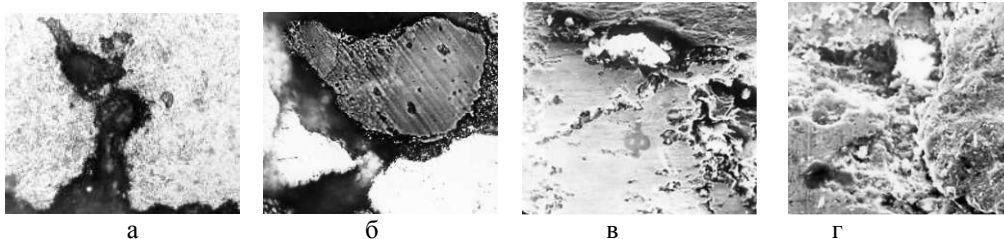
Рис. 1. Зарождение коррозионных повреждений на неметаллических включениях (Fe,Mn)S (а, з), MgO·Al 2 O 3 (б), MnO·SiO 2 (в) в сталях ШХ15 (а - в) и ШХ15Г (з) после испытаний на малоцикловую усталость в 5%-ном водном растворе NaCl (а, в, з) и 1%-ном водном растворе H 2 SO 4 (б): х600
