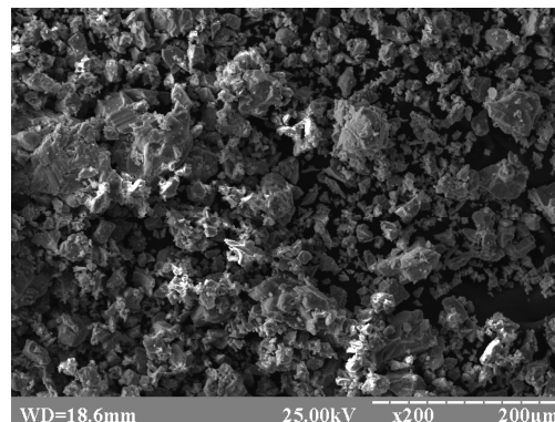
Рис. 3 – Частицы порошка гидрированного титана губчатого / Particles of hydrogenated titanium spongy powder
