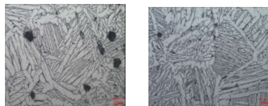
Рис. 5 – Микроструктура спеченного титана, полученного методами ПМ:
