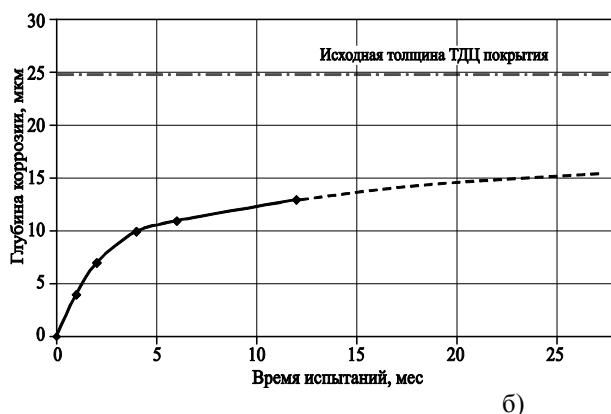
Рис. 2. Кинетика коррозии цинковых покрытий в условиях, имитирующих слабоагрессивную промышленную атмосферу с SO_2 (ГОСТ 26294-84) (а) и зависимость глубинного показателя коррозии диффузионного цинкового покрытия при ускоренных испытаниях в камере влажности с SO_2 и последующего периодического погружения в 0.001 н. раствор H_2SO_4 от времени испытаний (б). (1 месяц испытаний соответствует ~ 1,2 годам натуральных испытаний) / Kinetics of zinc coating corrosion in the conditions simulating lightly corrosive industrial atmosphere with SO_2 (GOST 26294-84) (а) and dependence of the depth index of diffusion zinc coating corrosion in accelerated tests in a humidity chamber with SO_2 and subsequent periodical immersion into 0.001 N solution of H_2SO_4 on the test duration (б). (1 month of tests corresponds to 1.2 years of full-scale tests)
