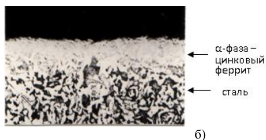
Рис.1. Микроструктура диффузионного цинкового покрытия, полученного в порошковых смесях (а) и \alpha -фазы – цинкового феррита (б), имеющего вид светлой полосы в структуре основного металла и являющегося переходной фазой от стальной основы к слою покрытия. (Растворимость цинка в \alpha -фазе при 250°C составляет 4,5 %) / Microstructure of diffusion zinc coating applied in powder mixtures (а) and \alpha -phase – zinc ferrite (б) having appearance of a light band in the base metal structure and being a transient phase from the steel base to the coating layer. (Zinc solubility in \alpha -phase is 4.5% at 250 °C
