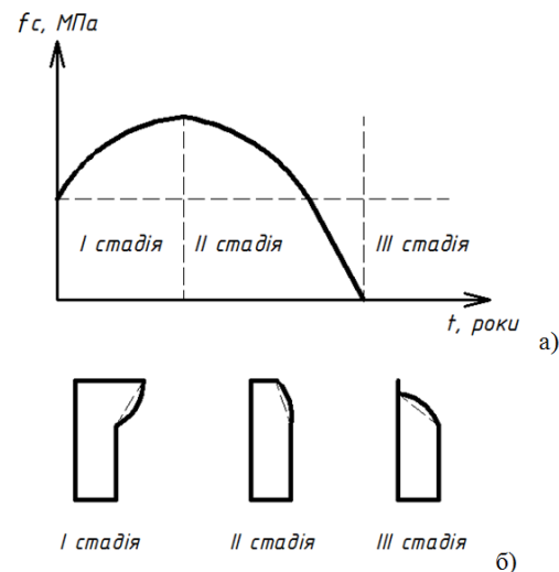
Рис. 1. Схема зміни міцності бетону при постійному впливі сульфатних розчинів / Scheme of changes durability of concrete at the constant influence of sulfate
