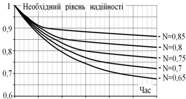
Рис. 3. Залежність інтенсивності зниження коефіцієнту готовності від рівня організаційно-технологічної надійності / The relationship between the level of organizational and technological reliability and reduction speed of readiness coefficient
