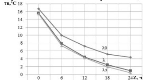
Рис. 4. Зависимость изменения температуры внутренней поверхности стенки при отключении системы теплоснабжения для II типа здания ( \rho = 1600 \text{ кг/м}^3 )
