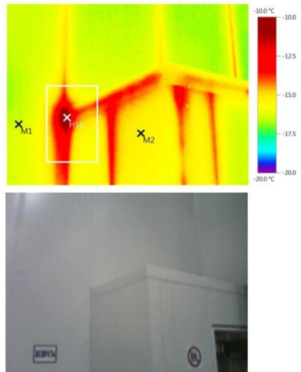
Рис. 3 Термическое изображение встроенного помещения в холодильной камере / Thermal image of embedded space in the refrigerator
