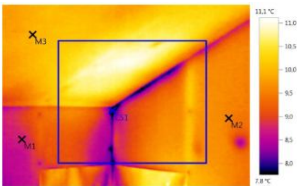
Рис. 1 Термическое изображение угла помещения мансардного этажа / Thermal image of the corner room on attic floor
