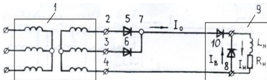
Рис. 1 Схема системы импульсного питания с двухфазным выпрямлением тока / Schematic diagram of a pulsed power supply system with two-phase current rectification
