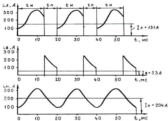
Рис. 2 Графическое представление токов в системе импульсного питания: i_L – ток в линии (ток в течение импульса); i_B – ток в цепи шунтирующего вентиля (ток в течение паузы); i_H – ток нагрузки; I_L, I_B, I_H – средние токи в линии, в шунтирующей цепи и в нагрузке / Graphics of instantaneous currents in the pulsed power supply system: i_L – line current (current during the pulse); i_B – current in the circuit of the shunt valve (current during the pause); i_H – load circuit current; I_L, I_B, I_H – average currents in the line, in the shunt circuit and in the load
