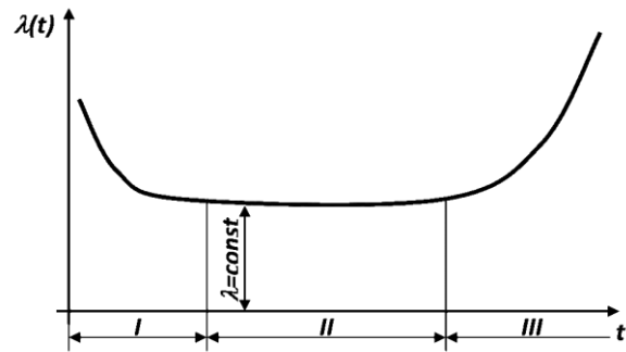
Рис. 1. Інтенсивність помилок оператора / The intensity of operator error
