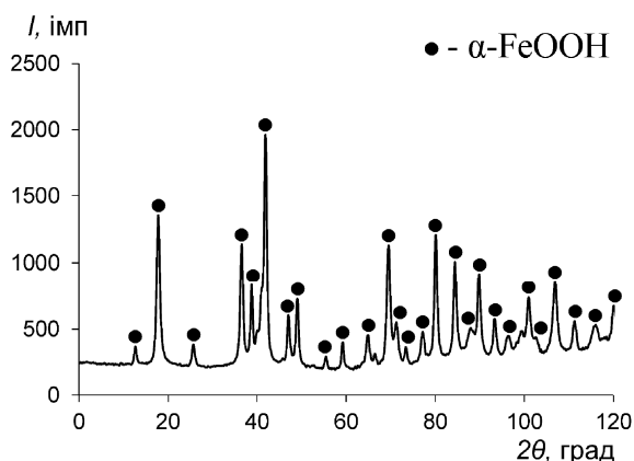
Рис. 1. Рентгенограма (а) і СЕМ-зображення (б) вихідного зразка НП \alpha\text{-FeOOH}
