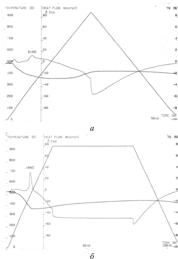
Рис. 2. Термогравиметрический анализ Ni-Co-Mn-Cu катализатора: а – до каталитических исследований, б – после каталитических исследований / Thermogravimetric analysis of the Ni-Co-Mn-Cu catalyst: a - before the catalytic studies, b - after catalytic studies
