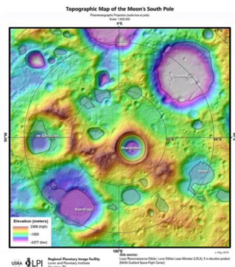
Рис. 5. Кратер Шеклтон, Південний полюс Місяця (Джерело: N + I). Опублікований атлас Південного полюса Місяця (Дата звернення – 11.4.2021). У ньому виявлені великі запаси льоду
