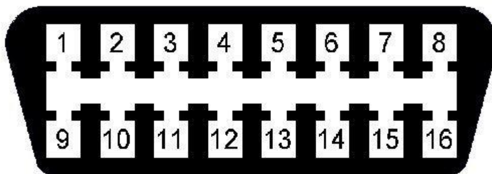
Рис. 3.1. Діагностичний роз'єм Opel Astra
