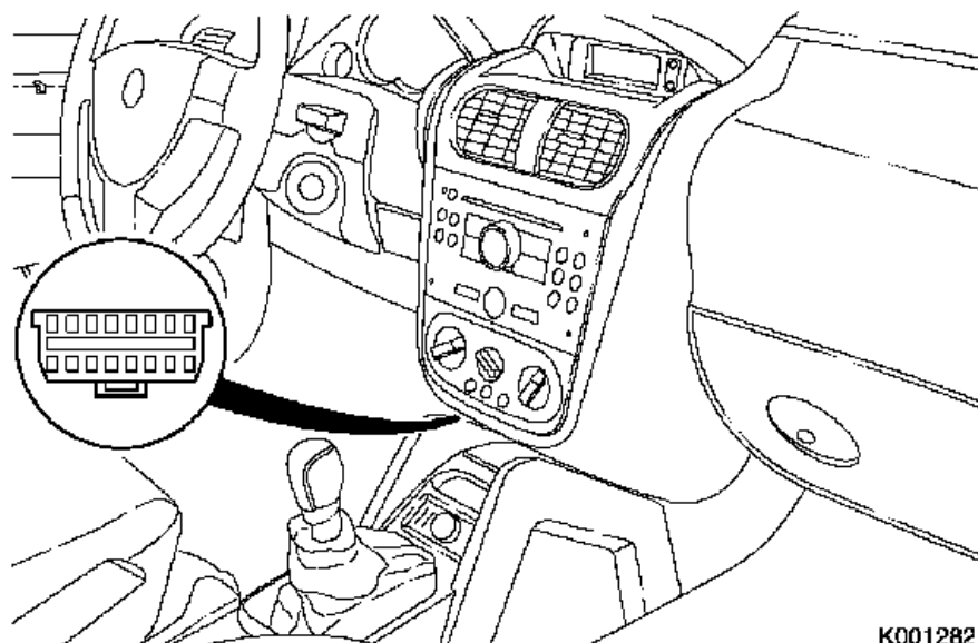
Рис. 3.6. Діагностичний роз'єм Opel Corsa C
