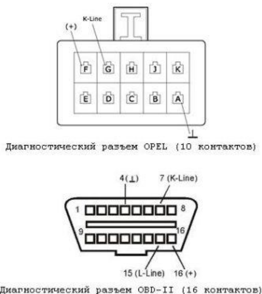
Рис. 3.2. Види роз'ємів , що використовує Opel
