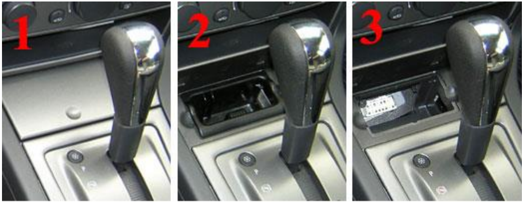
Рис. 3.9. Діагностичний роз'єм Opel Vectra C
