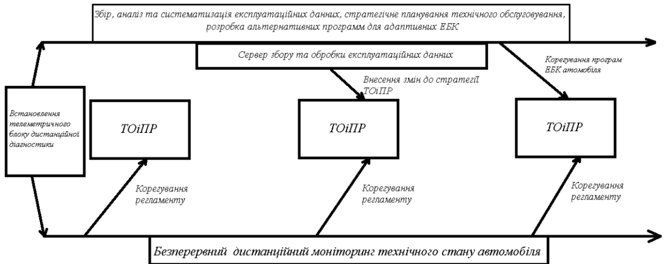
Рис. 4.4. Принциповий алгоритм і схема інтеграції процесів дистанційної електронної діагностики та аналізу експлуатаційних умов
