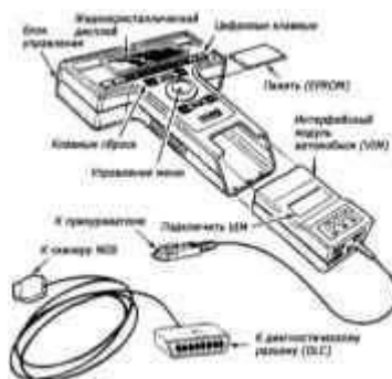
Рис. 3.14. Сканер типу Actron Scantool
