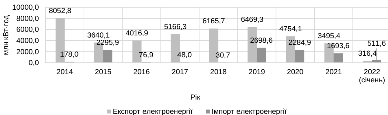
Рис. 4. Експорт та імпорт електроенергії з/до об'єднаних енергетичних систем України
